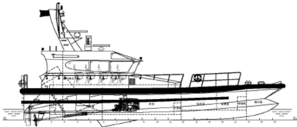
主甲板
