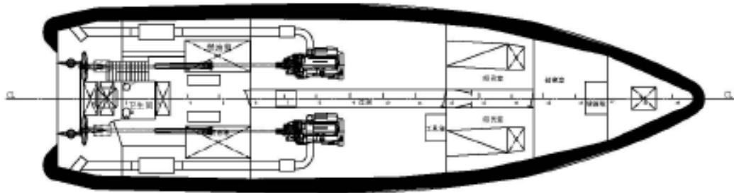
船底
